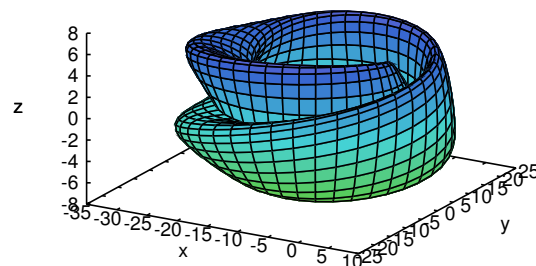
Parametric function
