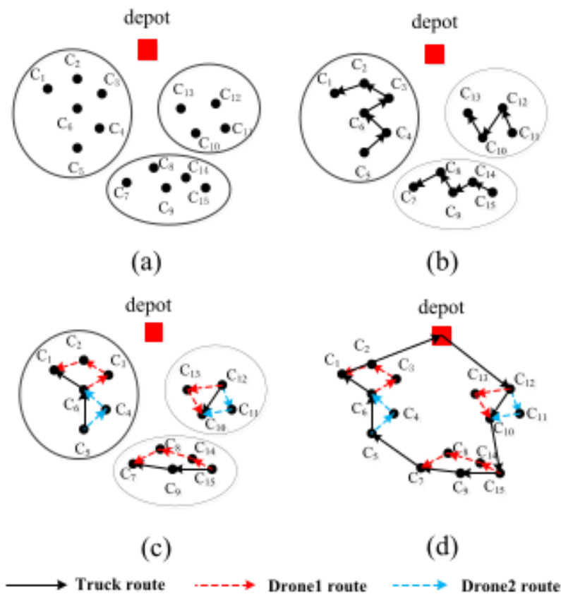
Obr. 6. a) Zákazníci rozdelení K-Means++, b) Konštrukcia trás vozidla, c) Konštrukcia letov dronov, d) Kompletná trasa vozidla [7]
