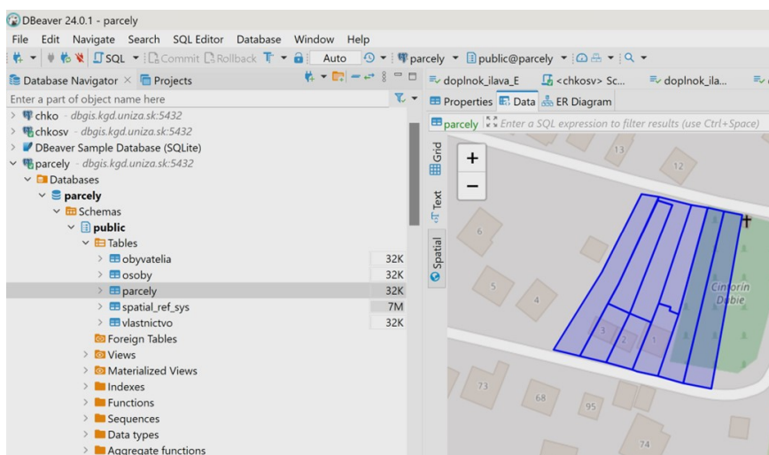
Obr. 2. Zobrazovanie priestorových dát priamo v prehliadači prostredia DBeaver
